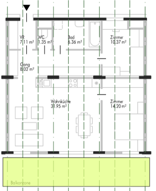
9 Achsen 79-80 m 2
