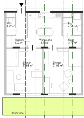
8 Achsen 69-70 m 2
