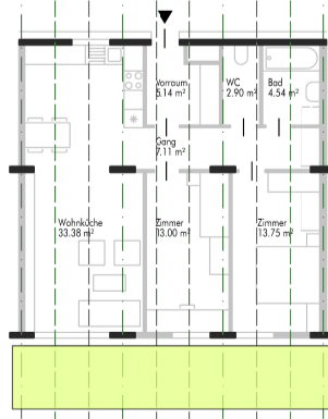
9 Achsen 79-80 m 2
